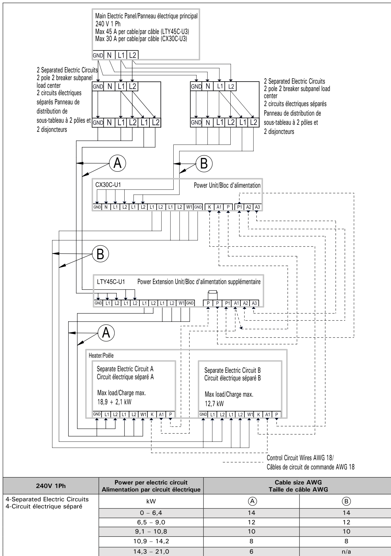
Figure 15. Connection of power extension unit LTY45C-U1 with control unit CX30C-U1 (240 V / 1Ph (Two separated electric circuits between power extension unit and heater). Heater with two built-in steamer units) Figure 15. Branchement du bloc d'alimentation supplémentaire LTY45-U1 avec centre de contrôle CX30-U1 (240 V / 1 Ph, deux circuits électriques séparés entre le bloc d'alimentation supplémentaire et le poêle). Poêle avec deux générateurs de vapeur intégrés)
